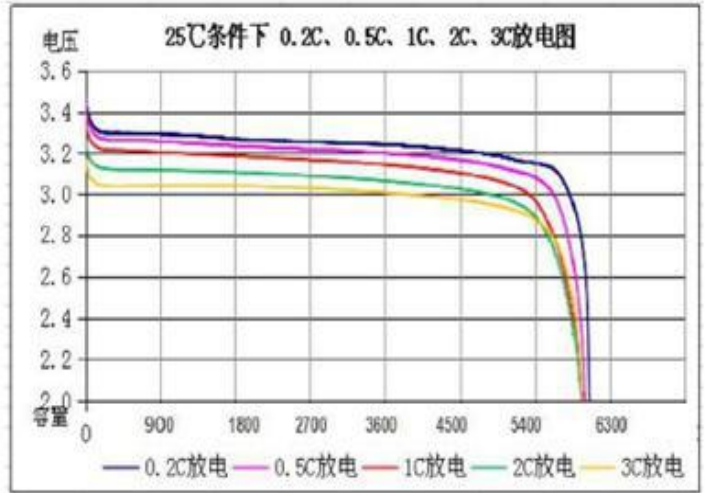
放电曲线图 Discharge discharge curve
