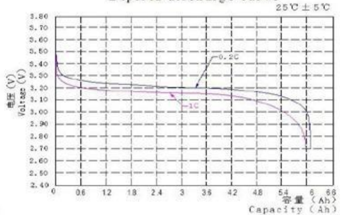
放电曲线图 Discharge discharge curve
